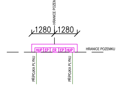
VZOR VYSAZENÍ PŘÍPOJKOVÝCH PILÍŘŮ 2RD
