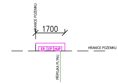
VZOR VYSAZENÍ PŘÍPOJKOVÝCH PILÍŘŮ 1RD
